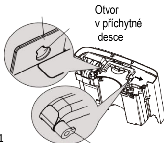
Rotační kolík v přichytné desce
